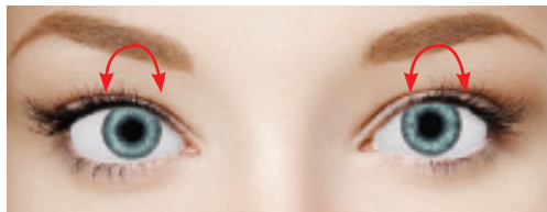
Torsional nystagmus.
