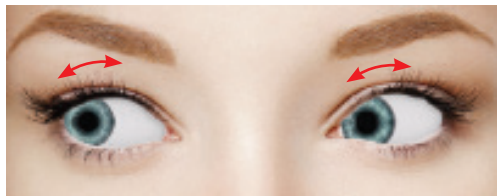
Horizontal nystagmus.
