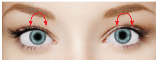
Torsional nystagmus.
